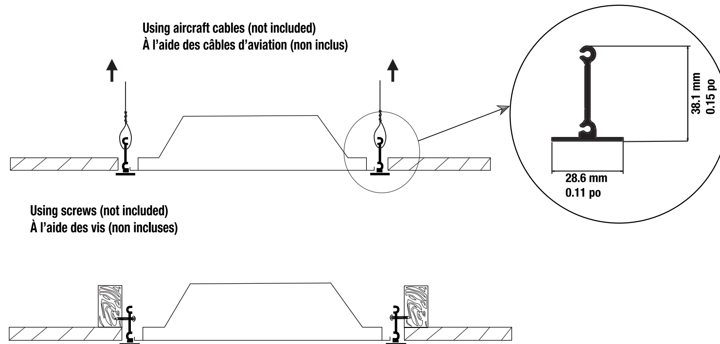
Fig. 3 MOUNTING METHODS / MÉTHODES DE MONTAGE
